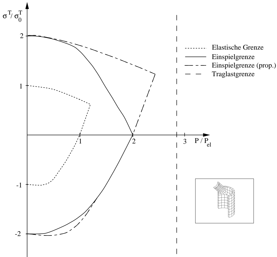
Bild 3: Interaktionsdiagramm des Rohrabzweigs
