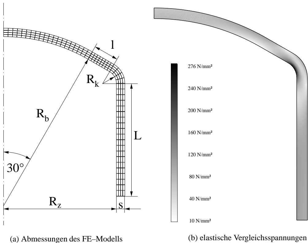
Bild 4: Abmessungen und VON MISES Vergleichsspannungen des FE-Modells
