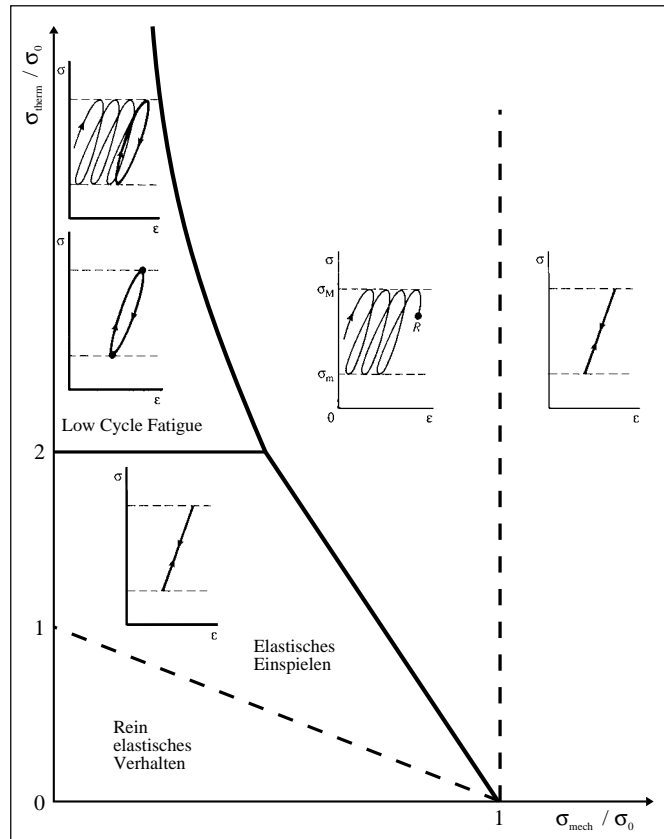
Bild 1: BREE-Interaktionsdiagramm für dünnwandige Rohre aus ideal plastischem Material. Es wird in dieser oder in modifizierter Form von verschiedenen Regelwerken genutzt [13].
