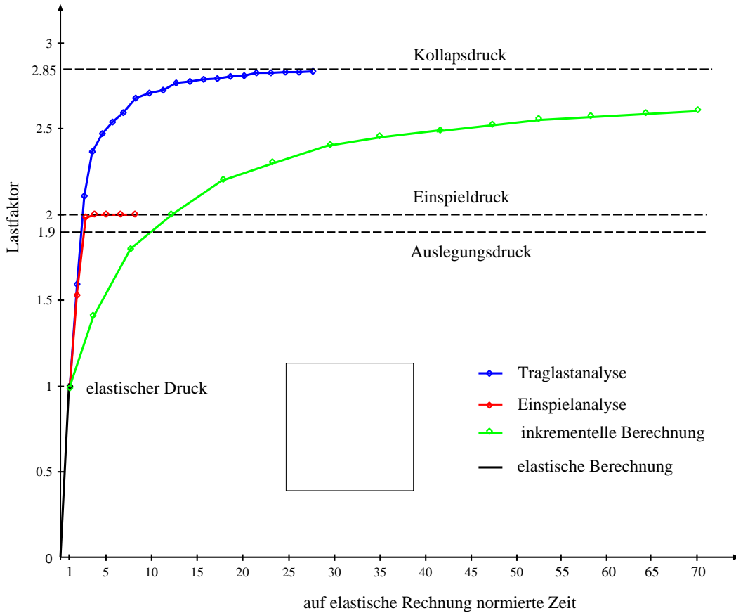
Bild 2: Rechenzeitvergleich für einen Rohrabzweig unter Innendruck
